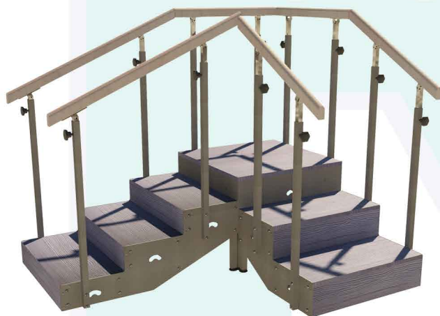
COMBINACIÓN DE LOS MÓDULOS DE 4 PELDAÑOS + DESCANSO + 3 PELDAÑOS EN ÁNGULO
