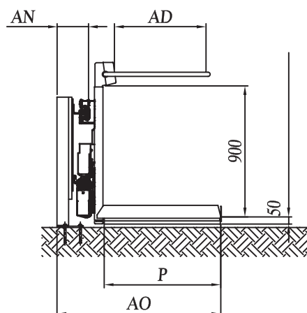
Plataforma abierta. Fijación con pies de soporte
